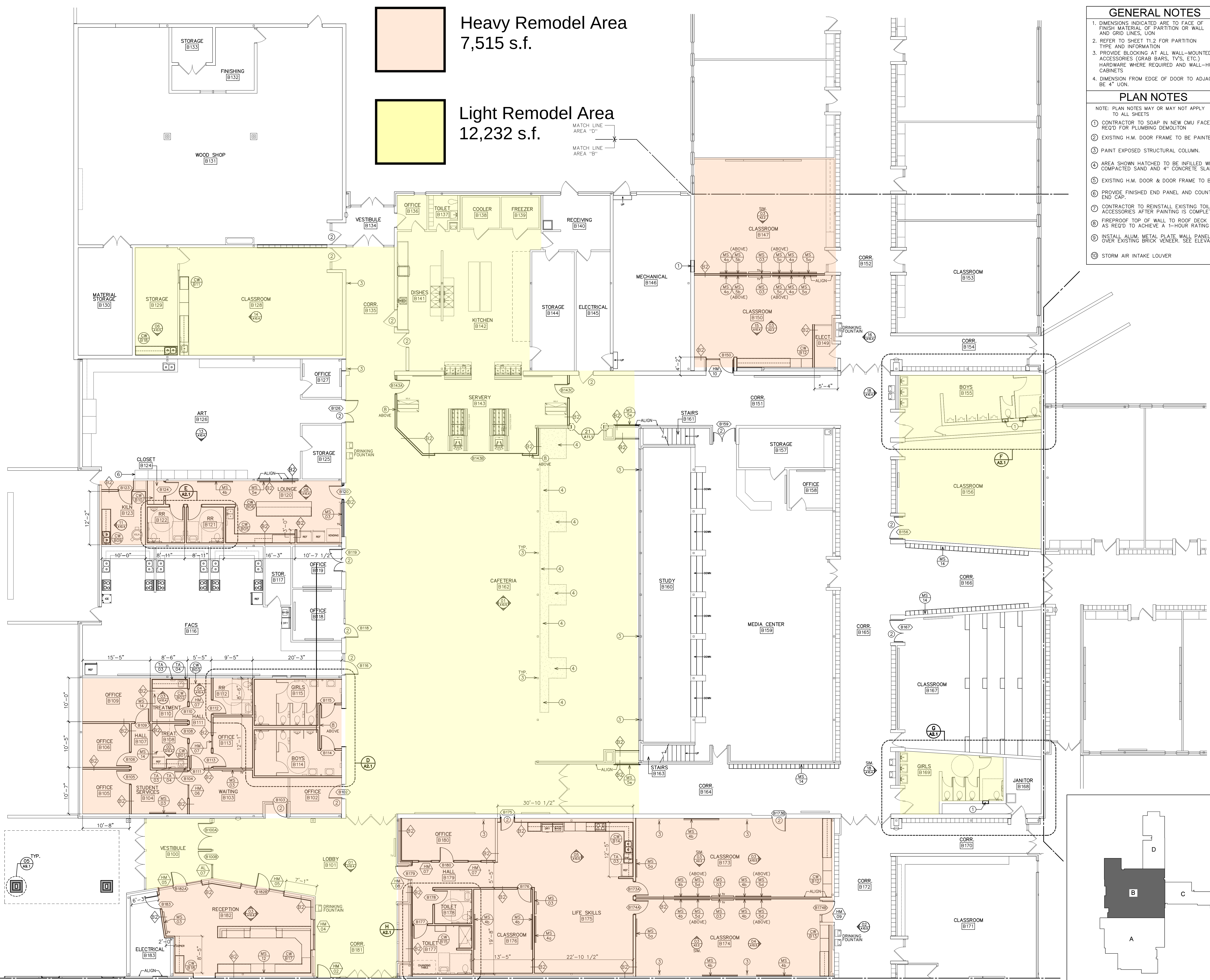
AREA 'B' FLOOR PLAN SCALE: 1/8" = 1'-0"
